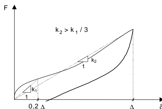
Figura C.5 - Requerimiento de rigidez para realizar análisis estático lateral equivalente
