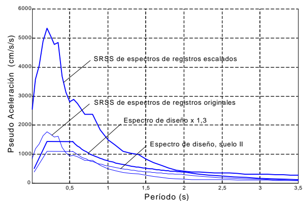
Figura C.19 - Amplificación de registros y combinación de componentes
