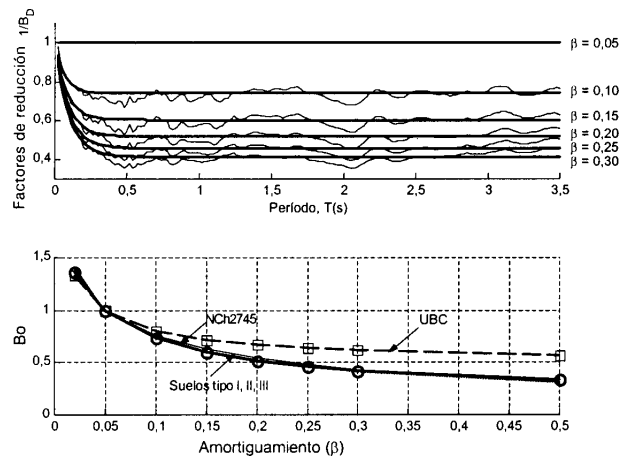
Figura C.15 - Factor de modificación de respuesta para suelo tipo II obtenido a partir de registros compatibles
