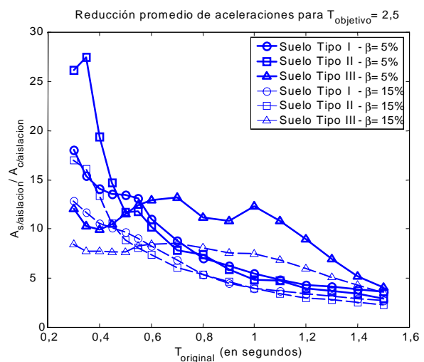
Figura C.4 - Reducción promedio de aceleraciones para estructuras aisladas de período objetivo 2,5 s, sometidas a los registros chilenos del terremoto de 1985 indicados en C8.4.2
