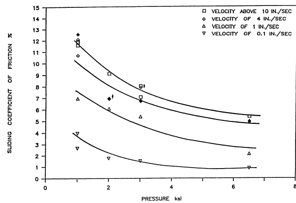
Figura C.14 - Variación observada de los coeficientes de roce \mu_{\text{mín.}} , \mu_{\text{máx.}} y \mu_s , como función de la presión de contacto (ver Anexo A, [26])
