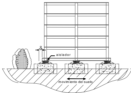
Figura C.2 - Modo fundamental de un edificio aislado
