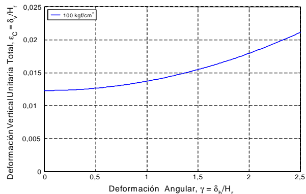
Figura C.11 - Descenso del aislador como resultado de la deformación lateral \gamma
