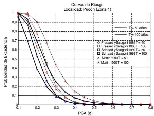
Figura C.1 - Probabilidad de excedencia de un nivel de aceleración máxima del suelo para tres sitios en suelo duro, en zonas sísmicas 3, 2 y 1, respectivamente, en lapsos de 50 y 100 años (Anexo A, [6, 14, 24])
