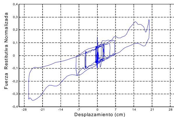
Figura C.22 - Efecto de la carga axial sobre la curva fuerza-deformación medida en un aislador FPS
