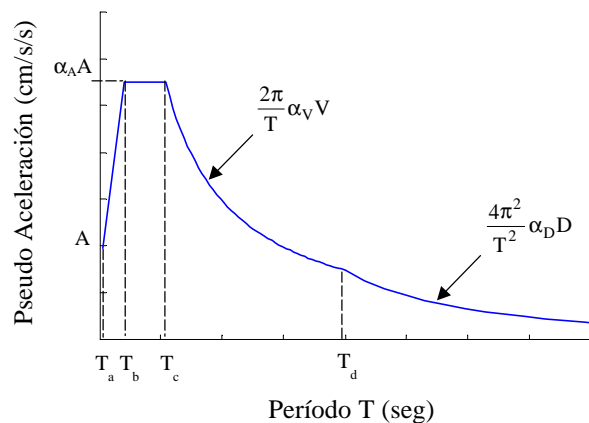
Figura C.17 - Definición del espectro de diseño de pseudo-aceleración
