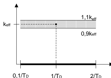
Figura C.20 - Definición de la zona de independencia de velocidad de carga para un aislador
