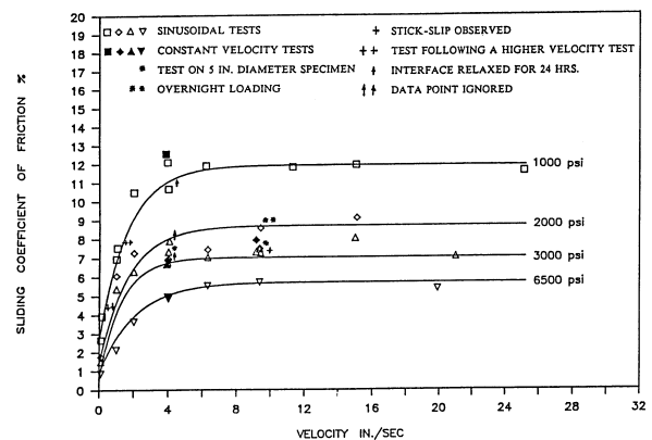
Figura C.13 - Variación del coeficiente de fricción dinámico \mu_d con la velocidad y presión de contacto (ver Anexo A, [26])
